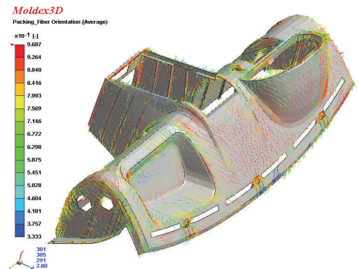
Genauere FEM-Lebensdauerberechnung mit präziseren lokalen Daten aus der 3D-Füllsimulation
